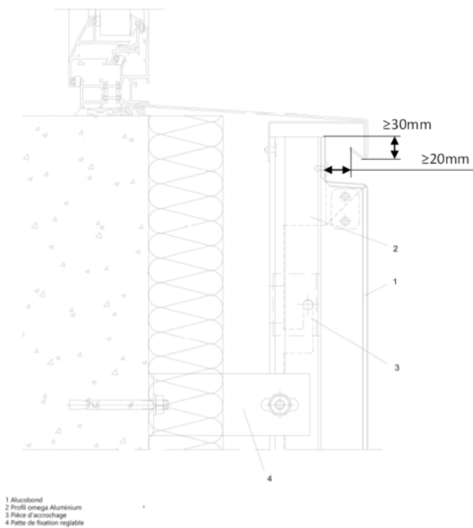
Figure 22– Raccordement de fenêtre en bas (Coupe verticale) (Système POB1)
