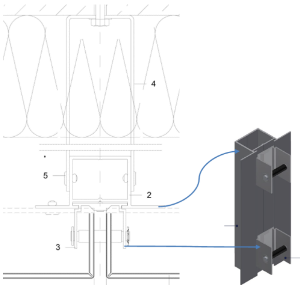
Figure 13 –Système POE1
