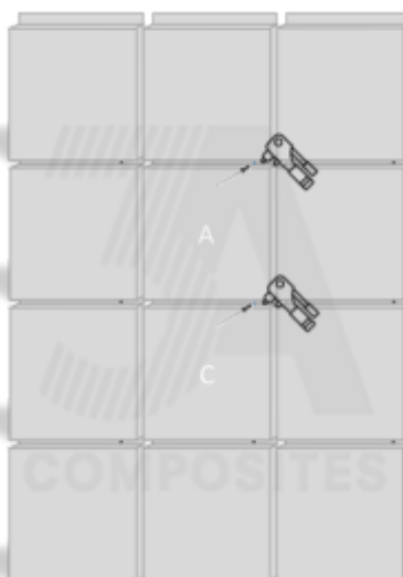
Figure 31 – Pas-à-pas de remplacement d'une cassette
