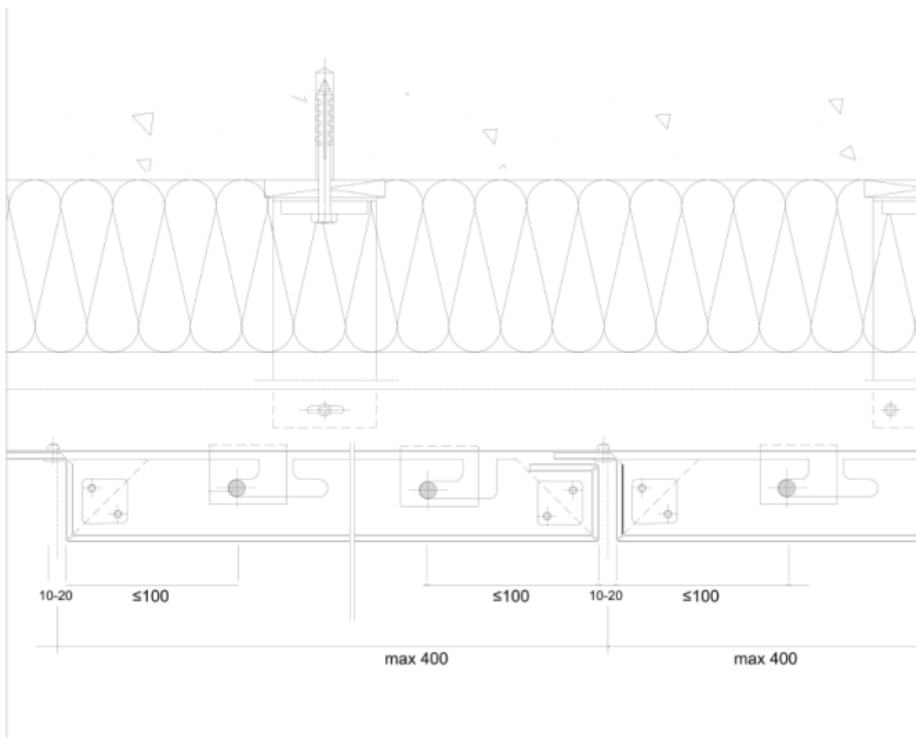
Figure 28– Cassette en sous-face (Coupe verticale)
