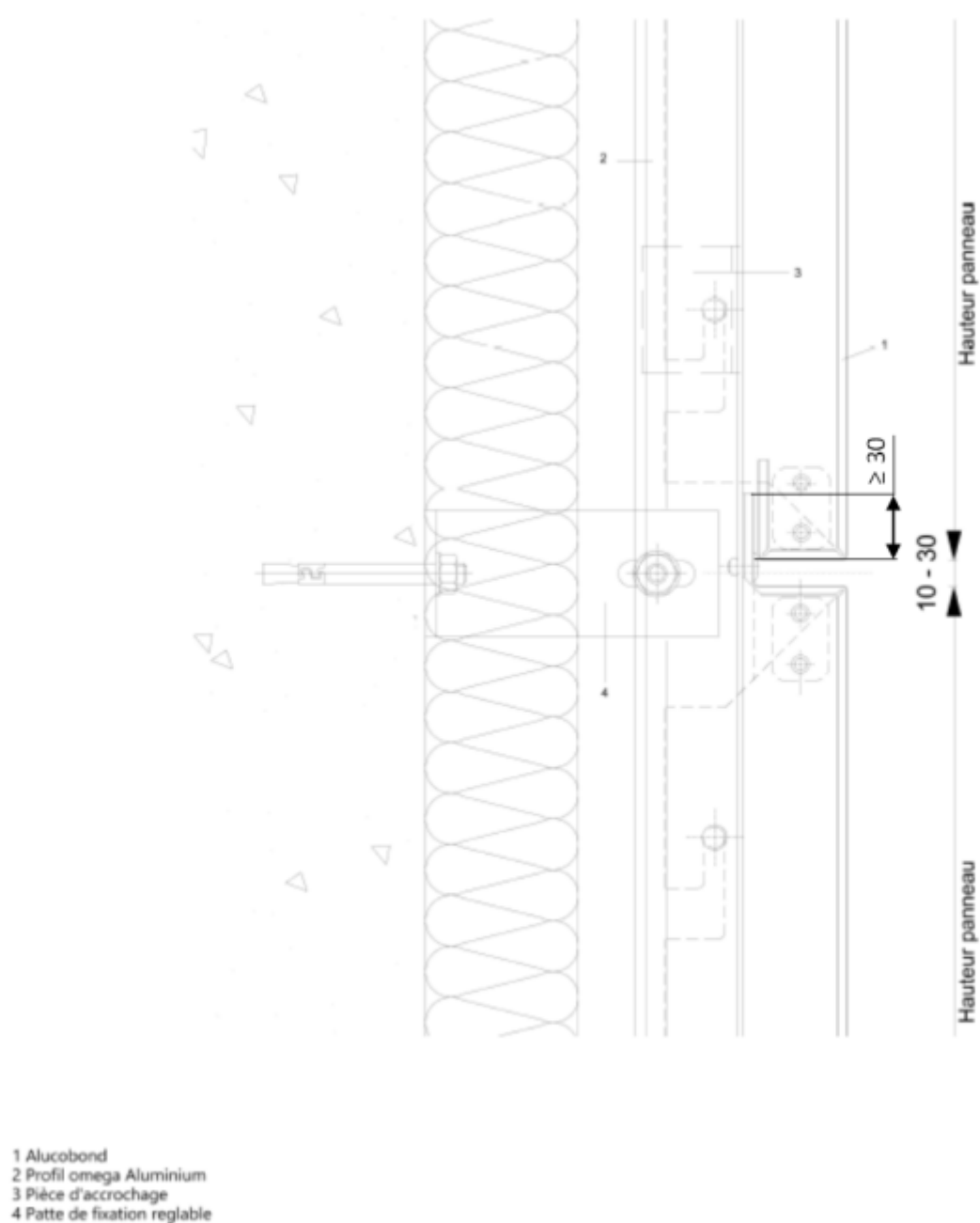
Figure 19 – Joint horizontal entre panneaux – Pose sur maçonnerie (Coupe verticale) (Système POB1)
