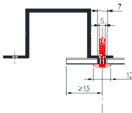
Vis de fixation (point coulissant)
