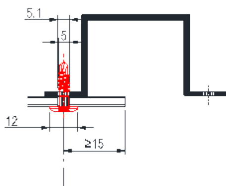
Vis de fixation (point fixe)
