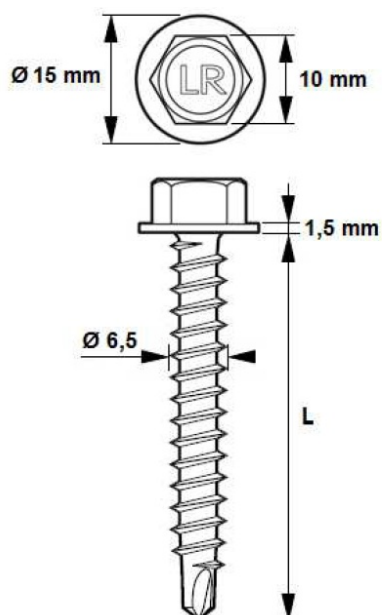
Figure 2c – Vis de fixation sur COB - Goldovis bois TH 10 de la Société Etanco
