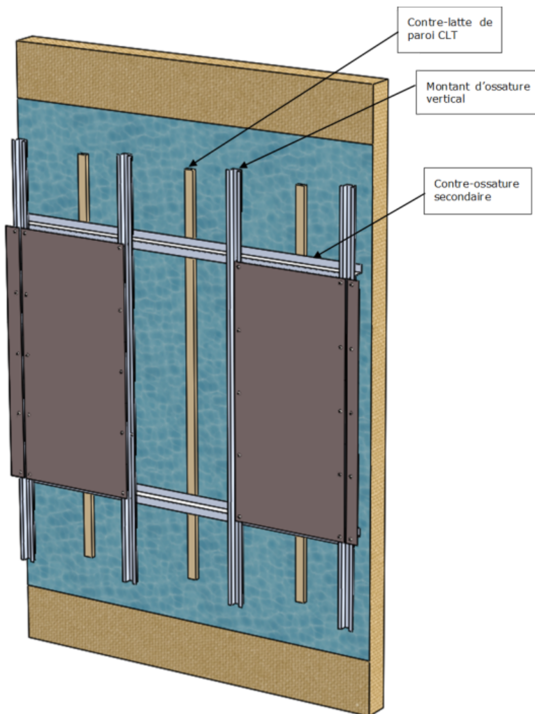
figure 4b – Principe de mise en œuvre du système LARSON riveté/vissé - Pose sur CLT
