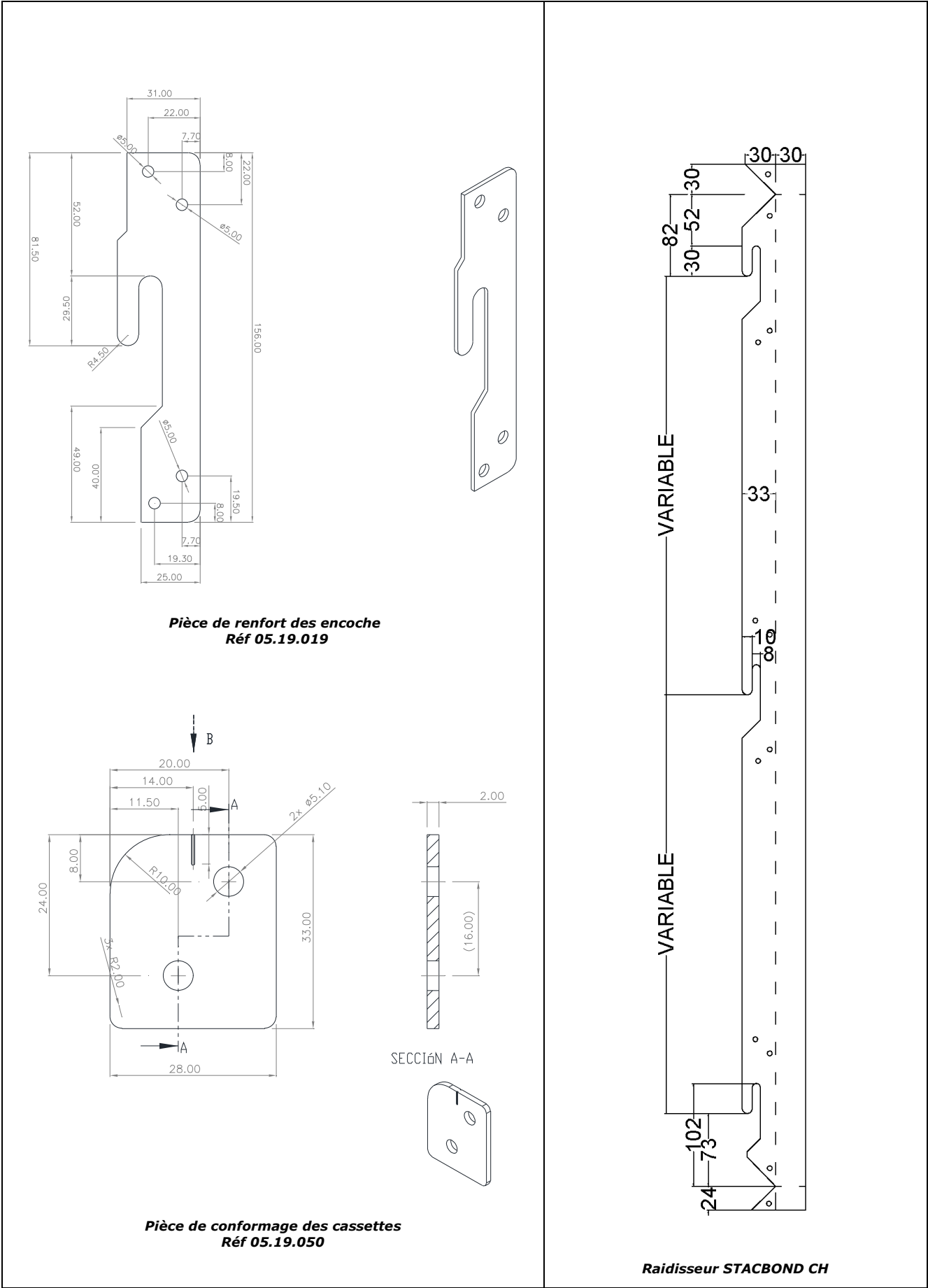
Figure 2c – Renforts latéraux et raidisseurs
