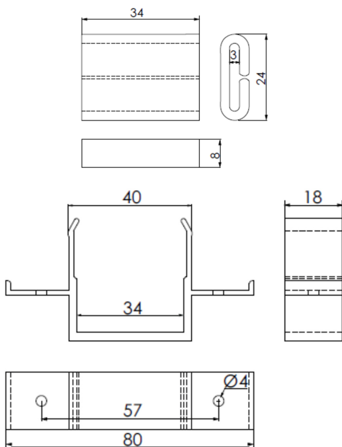
Figure 4 – Patte-agrafe réf. 05.19.013
