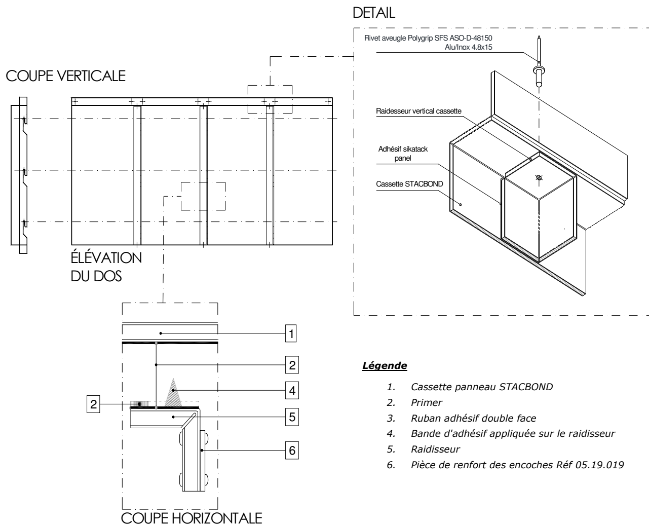
Figure 2d – Raidisseur mis en œuvre retours latéraux
